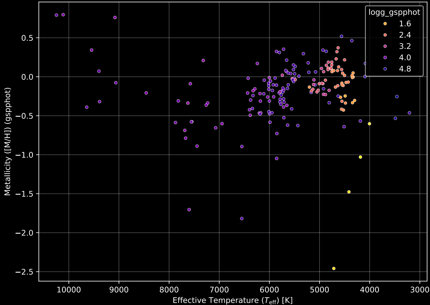
APOGEE DR17 Field: [CVZTILE_098+19_btx] Stellar Population Parameters (n= 178)
